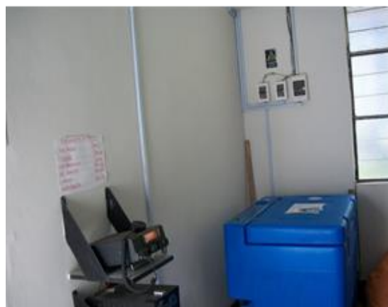
Fotos: Sistemas fotovoltaicos para iluminación, refrigeración y radio comunicación en los puestos de salud de Ternique y Los Ranchos
